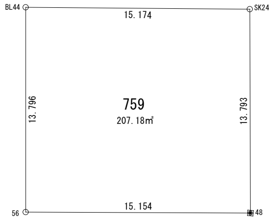
求積図 S=1/250
