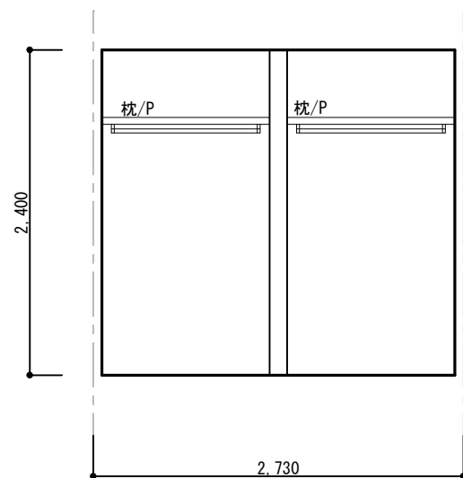
WIC
