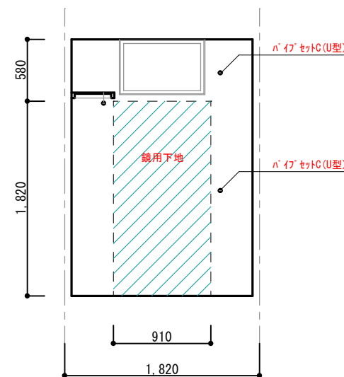
WIC
