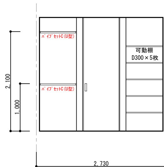
WIC
